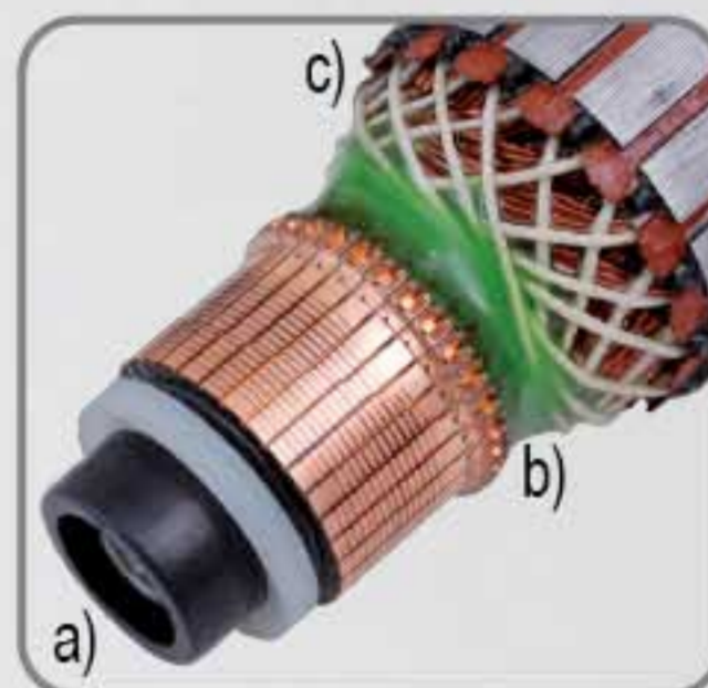
a) Sellos de neopreno en rodamiento, b) aislamiento epóxico en embobinado 100% cobre, c) malla de tela que brinda protección adicional al rotor contra residuos y partículas de metal.
