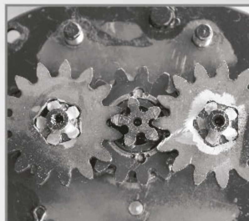
Caja de engranes fabricada en acero templado.
